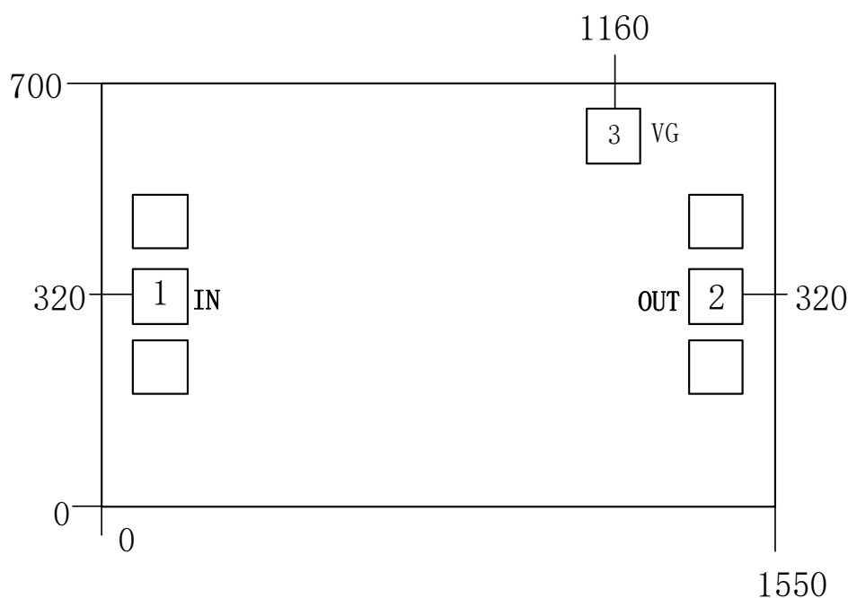
芯片端口图 (单位: \mu\text{m} )
